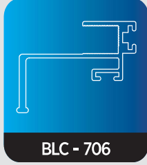
Cam Balkon Sürme Tutmalı Çekme Profili
