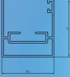
N1 Yan Profil (Yan-Alt Profil)
