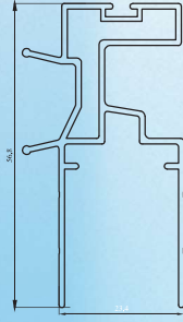
N1 - N2 Kayar Profil (Ara Profil)
