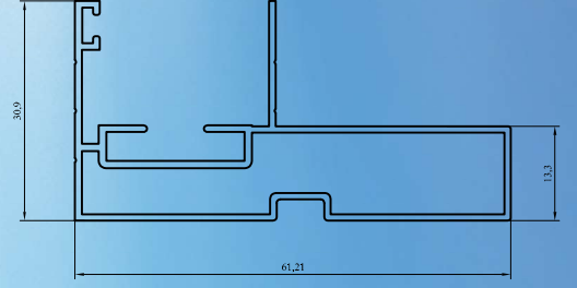
N2 Yan Profil (Yan-Alt Profil)
