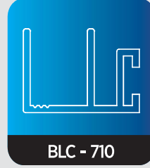
Cam Balkon Sürme Fitilli Cam Ara Kapatma Profili
